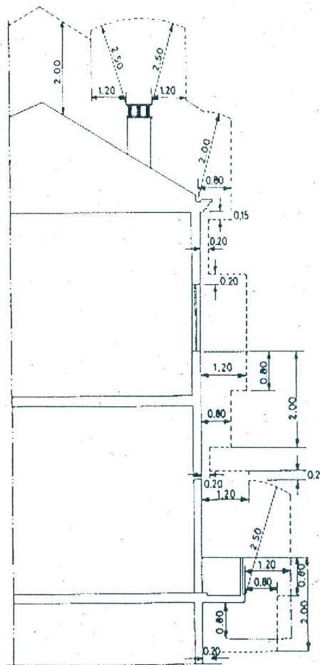
Figura 6: Figuras ilustrando a zona de protecção definida no n.º 1
