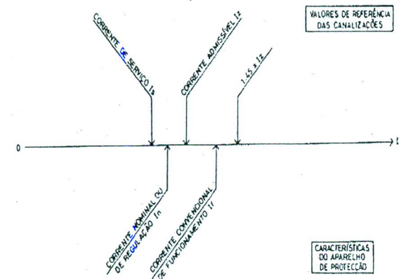
Figura 7: Esquema do funcionamento das protecções contra sobrecargas
